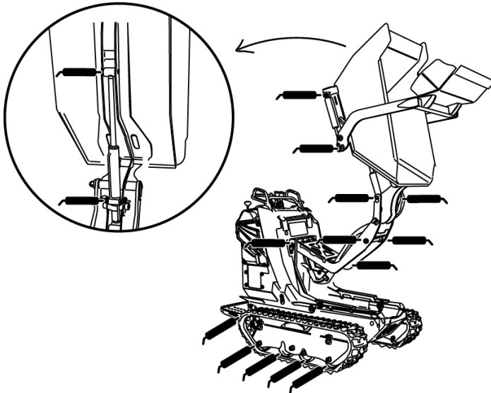
fig. 55 – Point de Graissage
