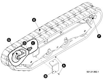
fig. 53 - Remplacement des chenilles
