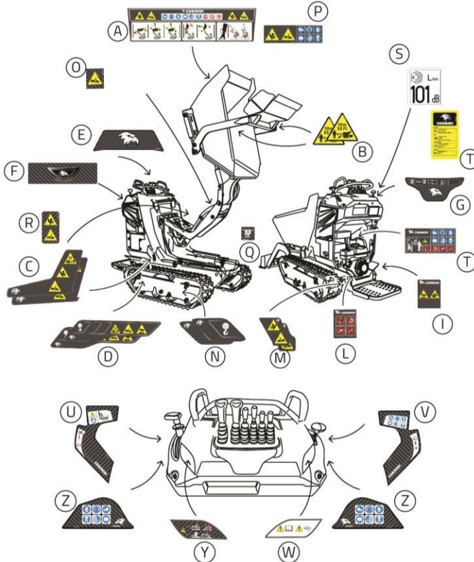
fig. 3 – Position des plaques de sécurité
