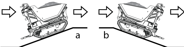
fig. 36 – a) marche en montée ; b) marche en descente
