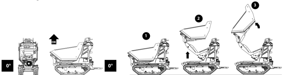
fig. 40 – Position pour le déchargement haut
