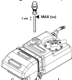
fig. 50 Niveau de l'Huile
