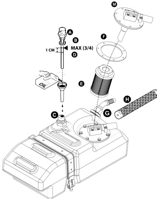
fig. 51 – Remplacement Huile et Filtres
