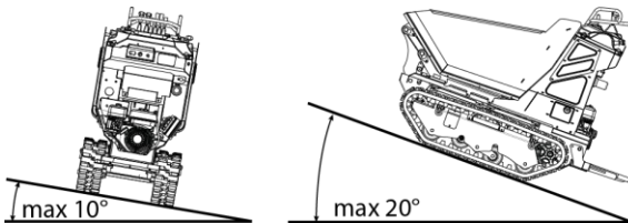
fig. 13 – Pentes maximales conseillées .
