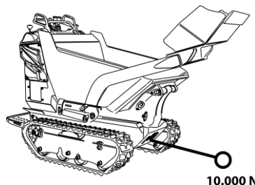
fig. 47 – Points d'ancrage pour la traction, avant et arrière
