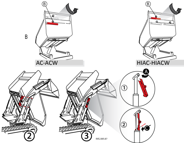
Abb. 3 – Hydraulikarmsperre
