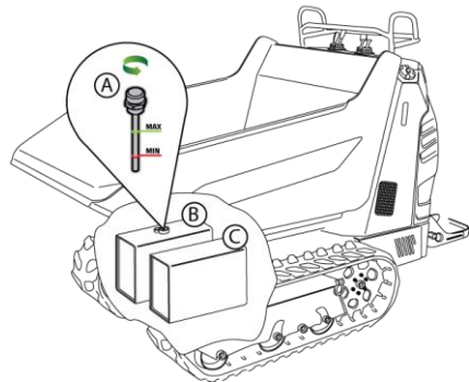
Abb. 34– Ölstand prüfen
