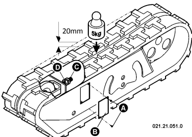
Abb. 35 - Einstellung der Spannung
