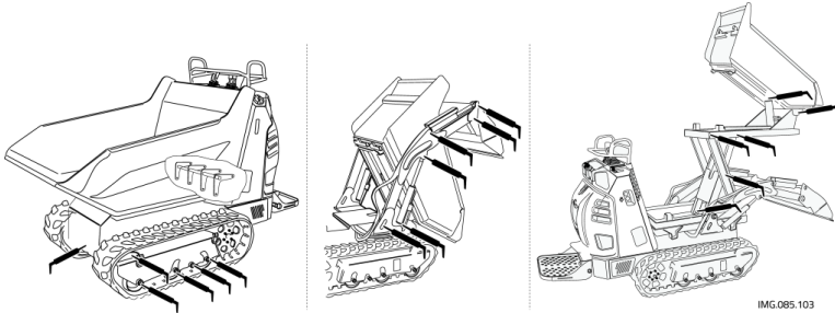
Abb. 56 – Schmierpunkte
