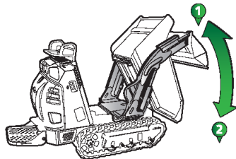
Abb. 14 – Kipphebel (oben) Hebel der Selbstladevorrichtung (unten)
