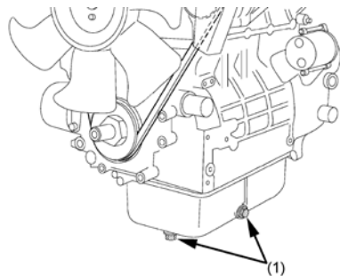
1. Ölablassschraube
