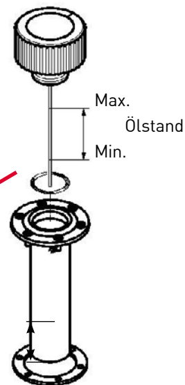
Einfüll-Belüftungsventil
