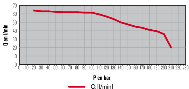
P/Q-ligne caractéristique circuit supplémentaire 1 TC35-2
