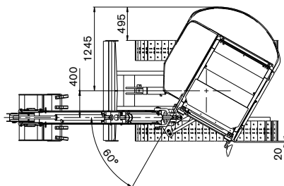
Fig. 1, 2 : Creuser sur toute la largeur de la machine
